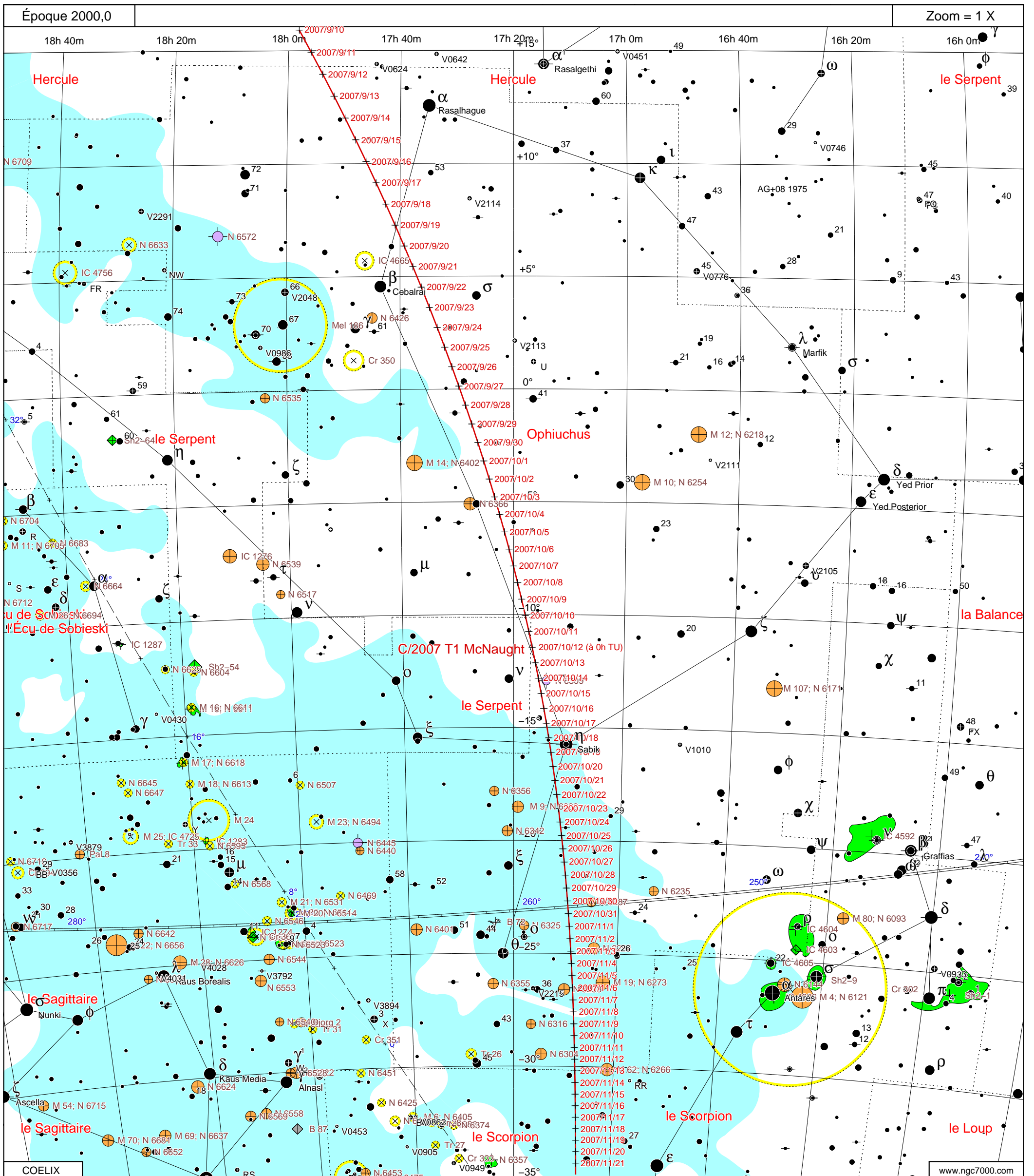
Magnitudes stellaires
